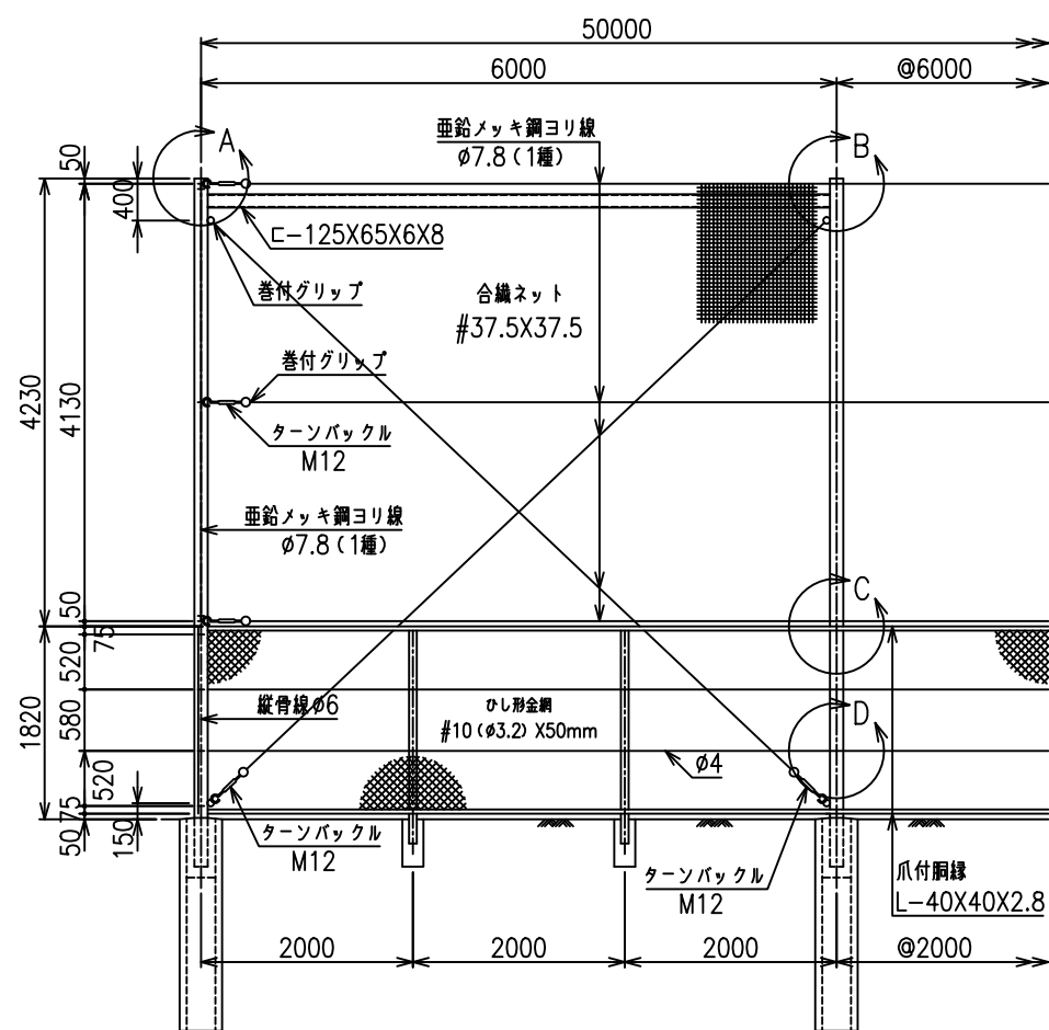
組立図 S=1/50
