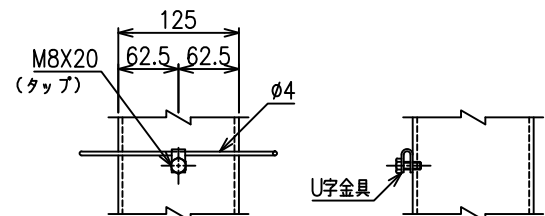
D部詳細図 S=1/5
