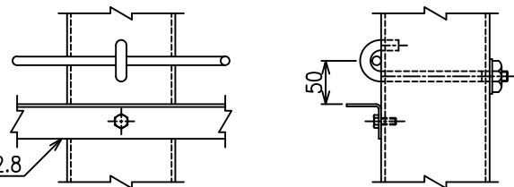
D部詳細図 S=1/5
