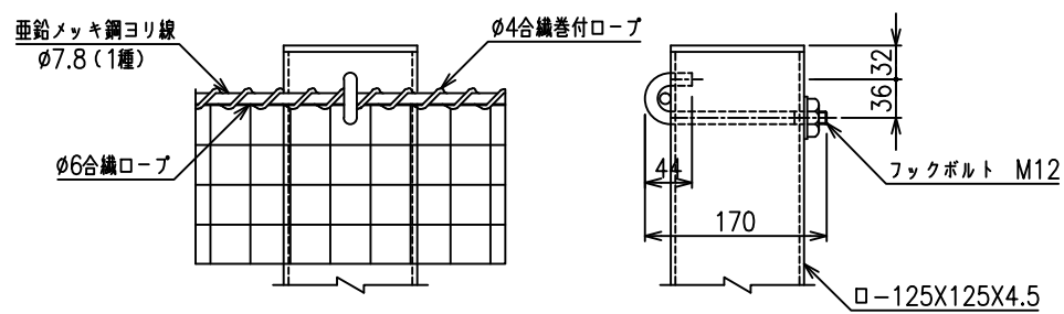
B部詳細図 S=1/5
