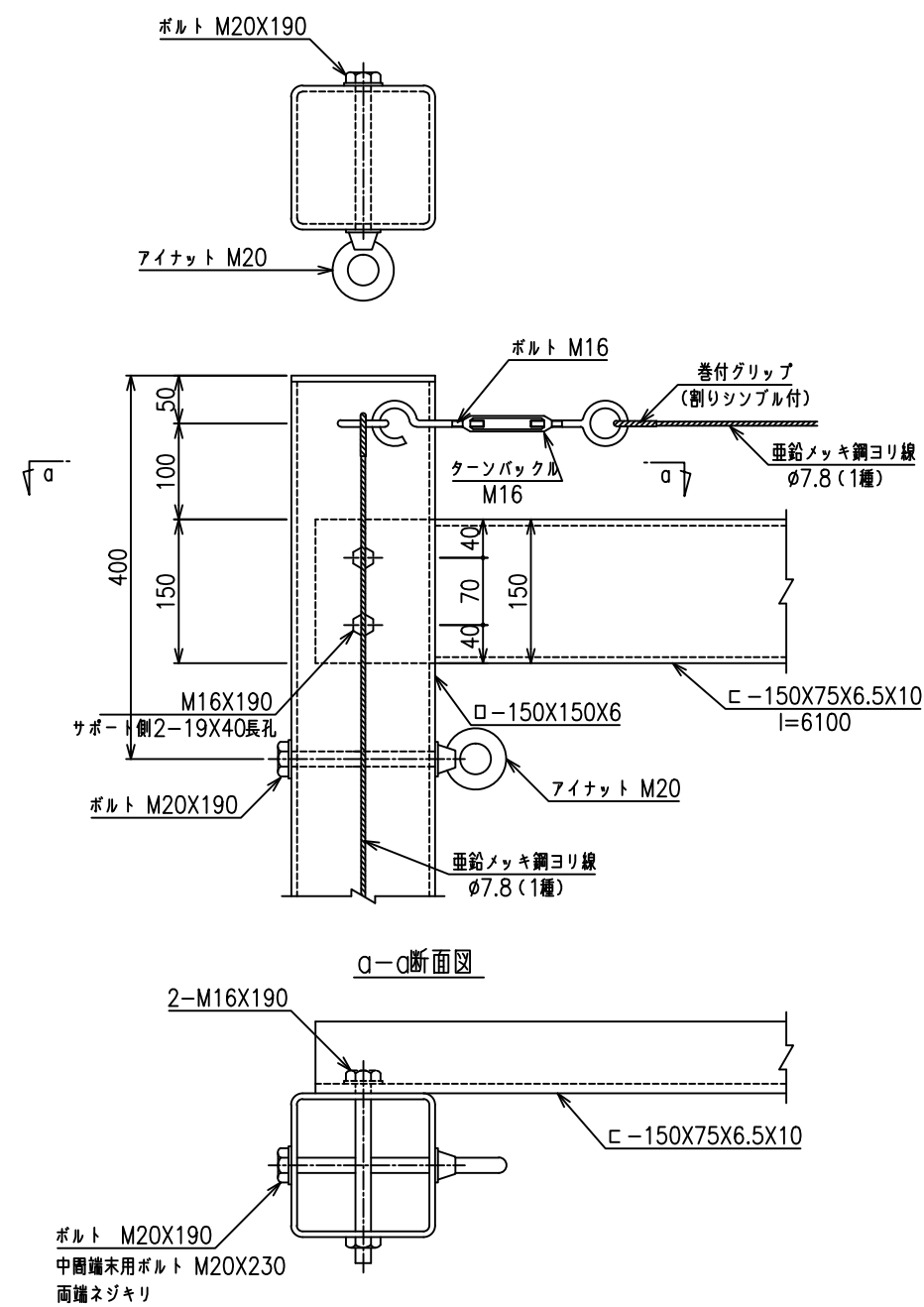
A部詳細図 S=1/5
