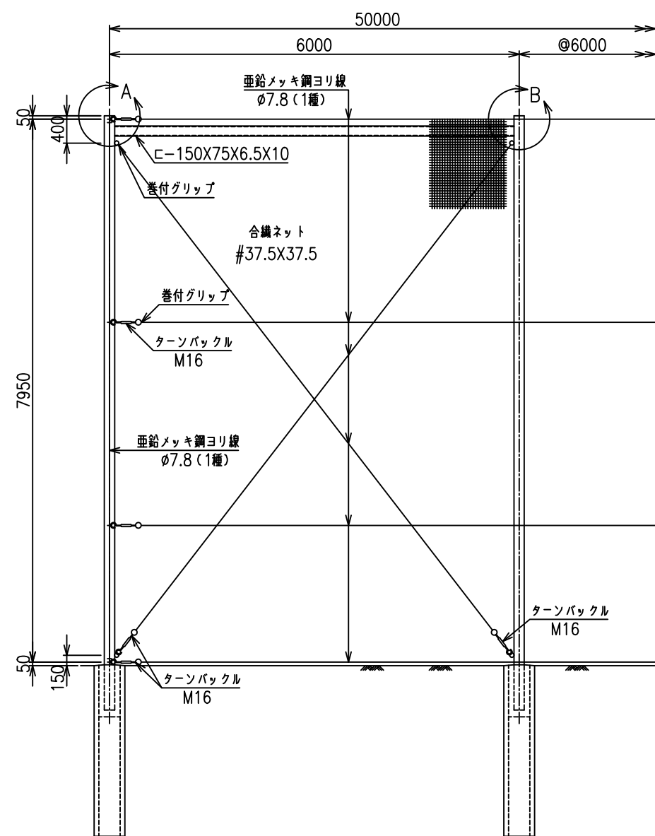
組立図 S=1/50
