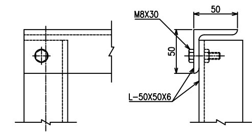
A部詳細図 S=1/2
