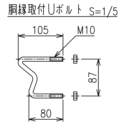
胴縁取付Uボルト S=1/5
