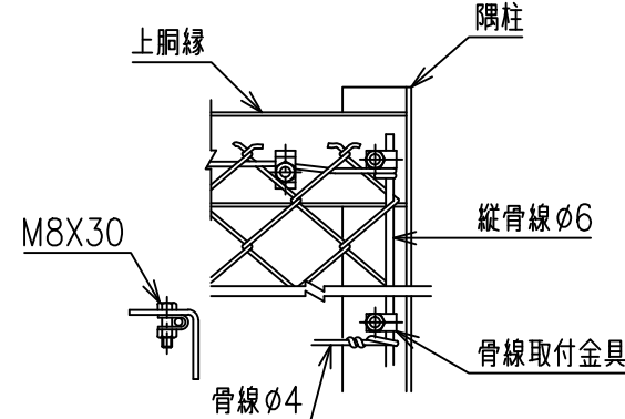
隅柱取付部 S=1/6
