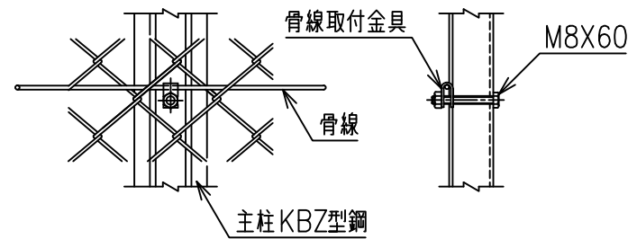
金網取付金具 S=1/2
