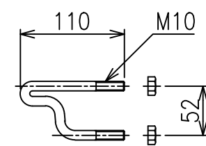
胴縁取付Uボルト S=1/5
