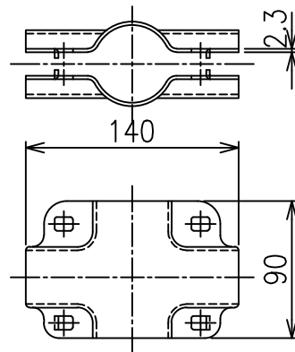
胴縁中間ジョイント S=1/4
