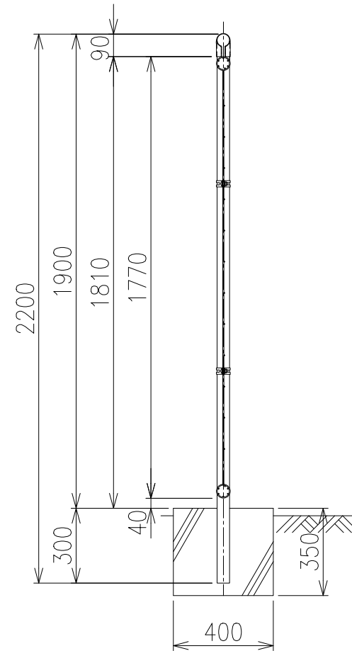
側面図 S=1/20
