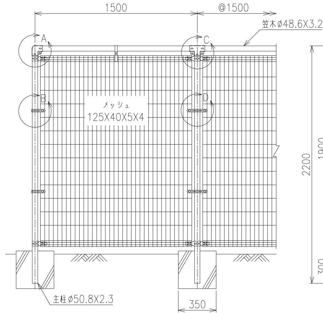
正面図 S=1/20
