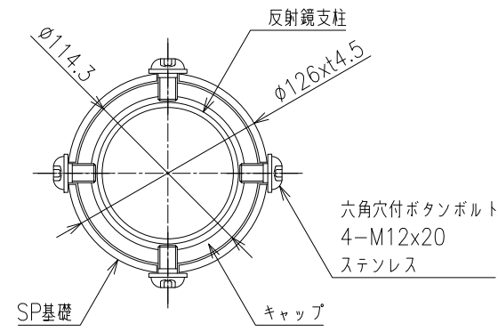
A-A詳細 S=1/3
