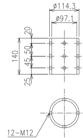
脱着式キャップ S=1/6 (φ89.1支柱用)
