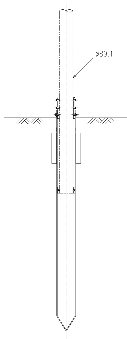
全体図 S=1/10
