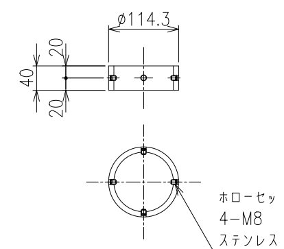
スペーサー S=1/6 (φ89.1支柱用)
