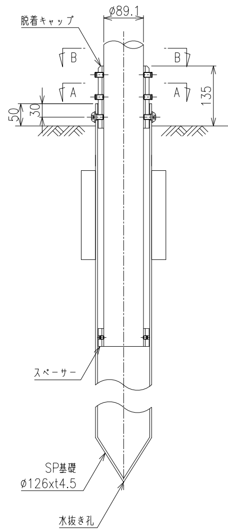
取付詳細図 S=1/6
