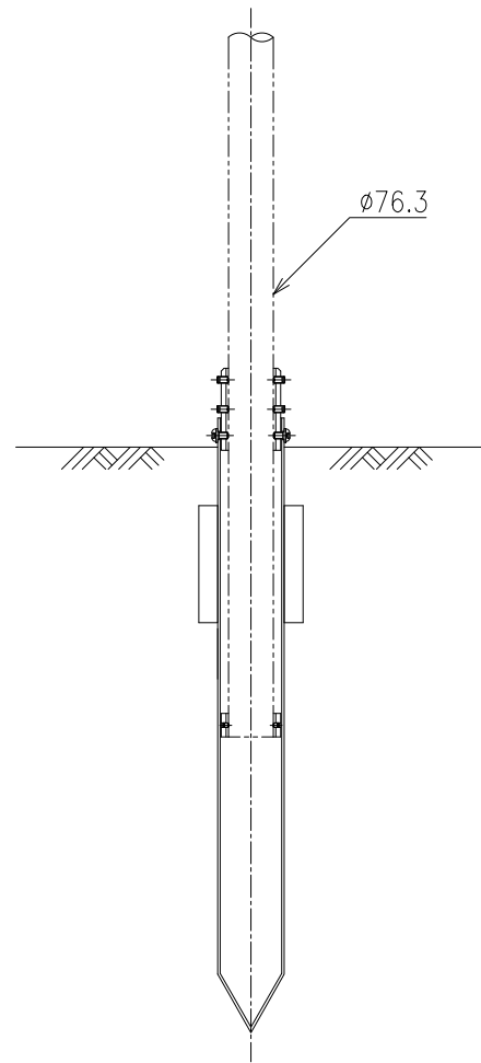
全体図 s=1/10
