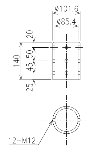
脱着式キャップ s=1/6 (φ76.3支柱用)
