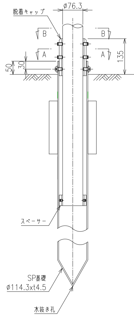
取付詳細図 s=1/6
