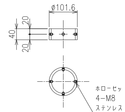
スペーサー s=1/6 (φ76.3支柱用)
