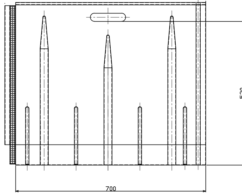
B断面
