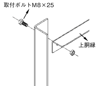
L型柱の場合
