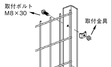
コーナー柱なしの張出しタイプ
