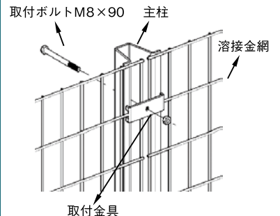
コーナー柱なしの張出しタイプ
