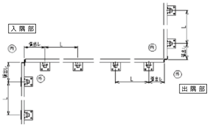
コーナー(張出しタイプ)
